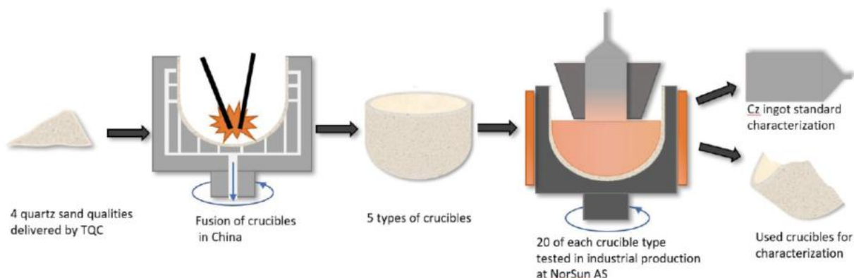
Figur V9. Illustrasjon av industriell skala forsøk gjennomført i SuSolTech. Bilde: SuSolTech sluttrapport
