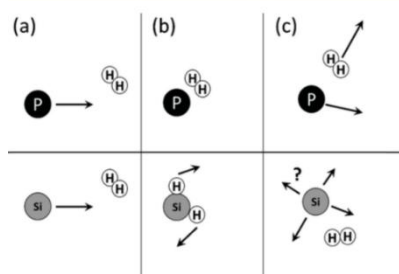
Figur V11. Illustrasjon av transport av P- og Si-atomer under forskjellige gasser (venstre). Typiske kollisjoner mellom P og Si og H 2 : (a) starttilstand, (b) nærmeste møte og (c) slutttilstand (høyre). Bilde: SuSoltech sluttrapport (Kilde: Arman Hoseinpour Kermani/NTNU og Stefan Andersson/SINTEF).
